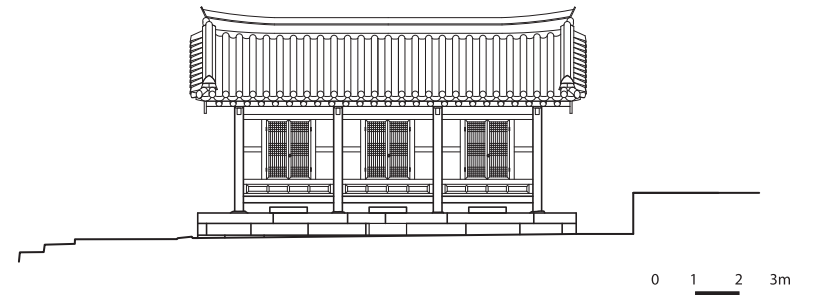
입면도
