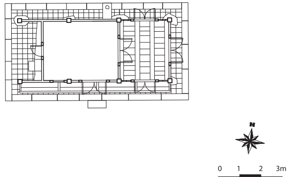
평면도
