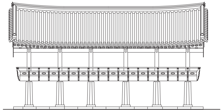
입면도
