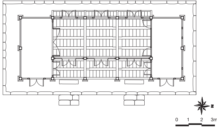
평면도
