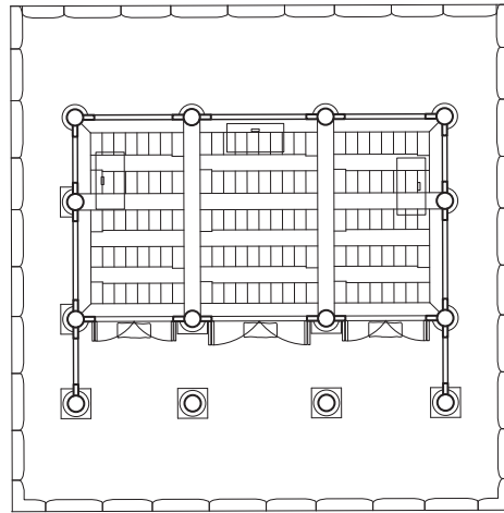
평면도
