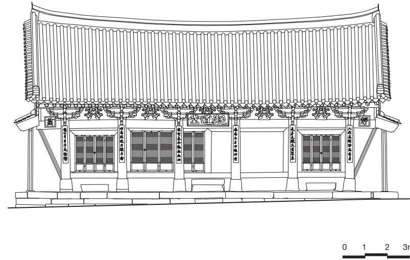
입면도
