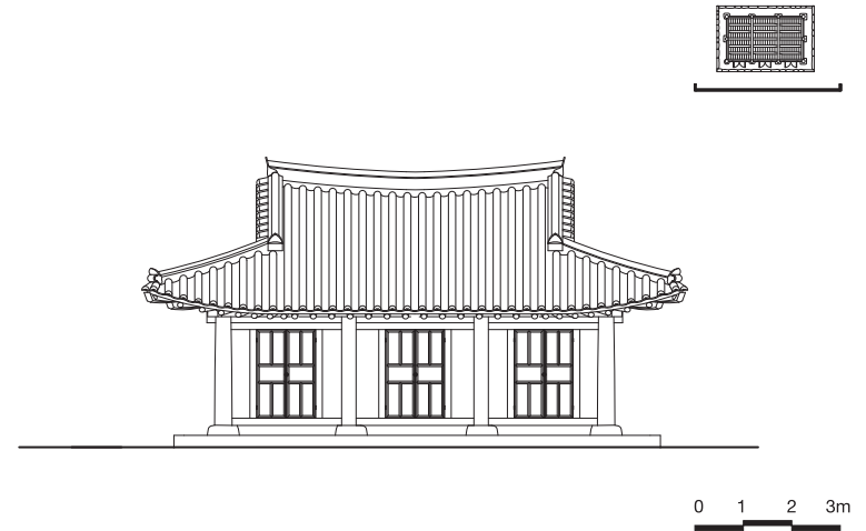
입면도
