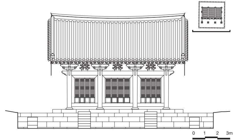
입면도
